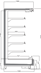
VECTO V3 2200 / 1090
