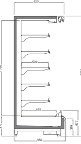
VECTO V3 2200 / 950
