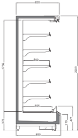
VECTO V3 2200 / 850
