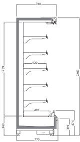
VECTO V3 2200 / 770
